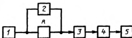
1 — генератор НЧ сигнала; 2 — вольтметр; 3 — измеряемая СЛ; 4 — номинальное сопротивление нагрузки; 5 — вольтметр
