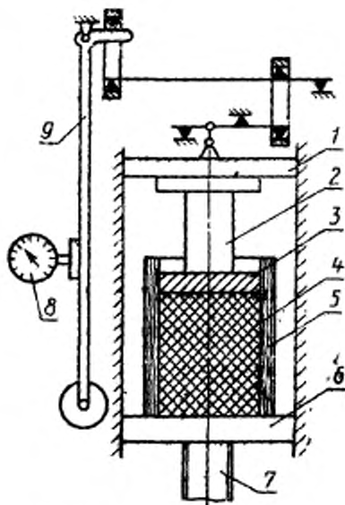
1 — верхняя плита; 2 — пуансон; 3 — диск; 4 — парафин; 5 — втулка; 6 — нижняя плита; 7 — шпигт; 8 — измеритель усилия; 9 — маятник
