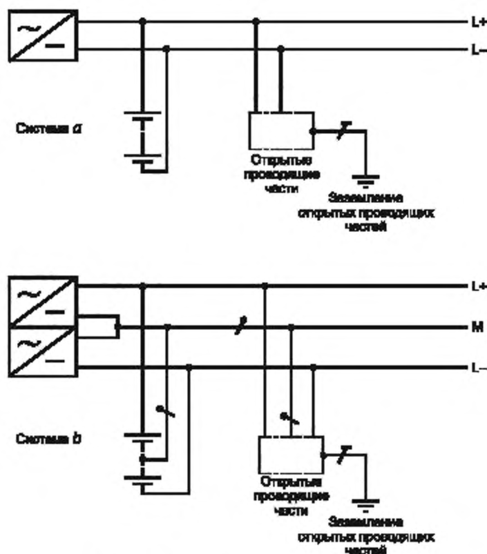
Рисунок 31К — Система IT постоянного тока
