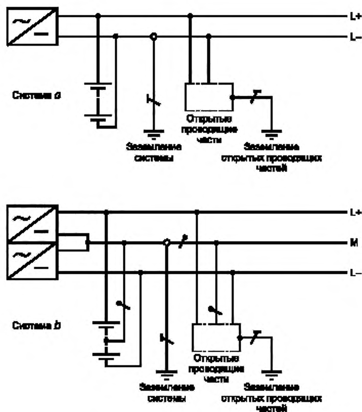
Рисунок 31J — Система TT постоянного тока
