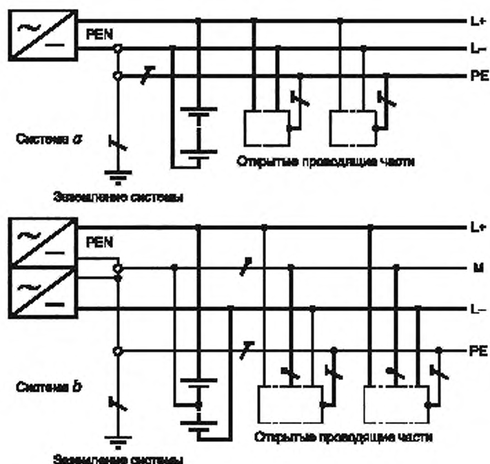
Рисунок 31F — Система TN-S постоянного тока
