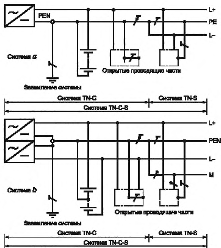
Рисунок 31Н — Система TN-C-S постоянного тока
