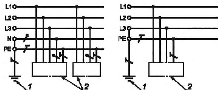
Рисунок 31А — Система TN-S (нулевой рабочий и нулевой защитный проводники работают отдельно)
