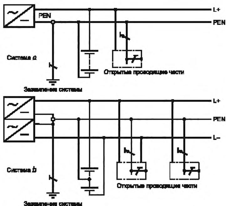
Рисунок 31G — Система TN-C постоянного тока
