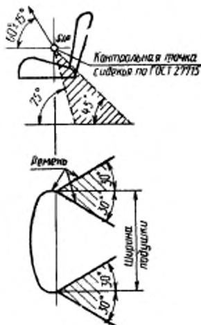
Места крепления ремней безопасности
