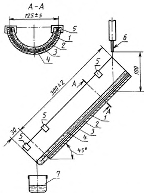
Контрольный прибор Размеры в миллиметрах
