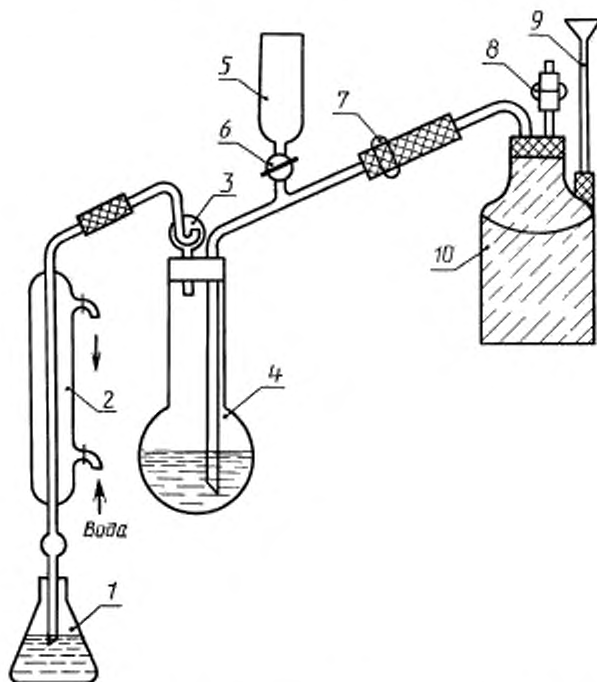
1 — приемная колба; 2 — холодильник; 3 — каплеуловитель; 4 — отгонная колба; 5, 9 — воронки; 6, 7, 8 — краны; 10 — парогенератор
