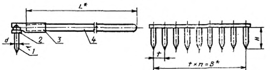
Вариант исполнения зуба
