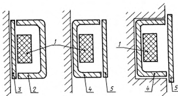
ОТКРЫТАЯ УСТАНОВКА
