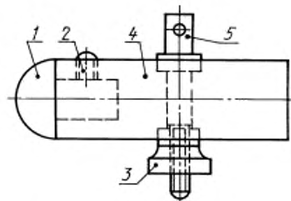
Материал детали поз. 1 — полиамид деталей поз. 2–5 — сталь
