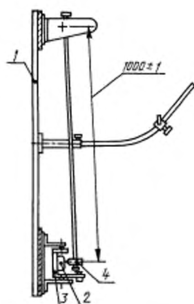
1 — опорная плита; 2 — образец; 3 — держатель образца; 4 — ударный элемент
