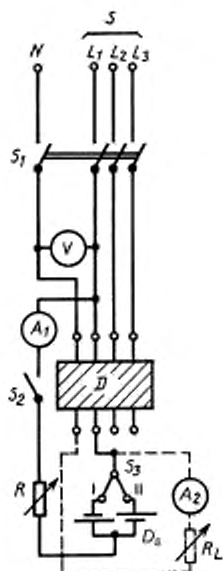
A_1 — амперметр постоянного тока; A_2 — амперметр переменного тока; D — испытуемое УЗО — Д; D_s — источник постоянного тока; R — регулируемый резистор; R_L — активная нагрузка; S — источник питания переменного тока; S_1 — многополюсный выключатель; S_2 — однополюсный выключатель; S_3 — двухполюсный выключатель на два направления; V — вольтметр
