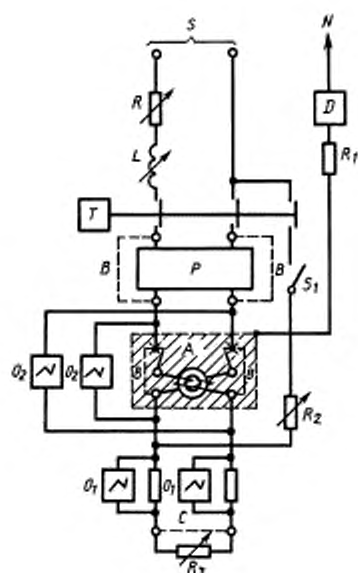
Рисунок 6 — Схема испытательной цепи для проверки правильности координации с аппаратом защиты от коротких замыканий и номинальной включающей и отключающей способности двухполюсного УЗО — Д без встроенной защиты от коротких замыканий в однофазной цепи
