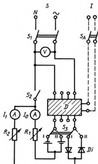
S — источник электрической энергии; I — независимая линия питания; V — вольтметр; A — амперметр; D — УЗО — Д, подвергается испытанию; Di — диоды; R_1 и R_2 — регулируемые резисторы; S_1 — многополюсный выключатель; S_2 — однополюсный выключатель; S_3 — двухполюсный выключатель на два направления; S_A — вспомогательный выключатель
