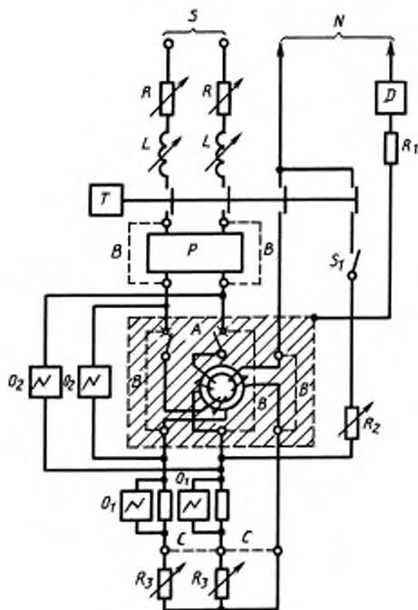
Рисунок 7 — Схема испытательной цепи для проверки правильности координации с аппаратом защиты от коротких замыканий и номинальной включающей и отключающей способности двухполюсного УЗО — Д с тремя путями прохождения тока без встроенной защиты от коротких замыканий в однофазной цепи со средней нейтралью
