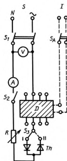
S — источник электрической энергии; I — независимая линия питания; V — вольтметр; A — амперметр (показывающий истинное действующее значение); D — УЗО — Д, подвергаемое испытанию; R — регулируемый резистор; S_1 — многополюсный выключатель; S_2 — однополюсный выключатель; S_3 — двухполюсный выключатель на два направления; S_4 — вспомогательный выключатель; Th — тиристоры
