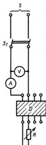
S — источник электрической энергии; S_1 — двухполюсный выключатель; V — вольтметр; D — испытуемое УЗО — Д; R — регулируемый резистор; A — амперметр
