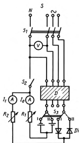
S — источник электрической энергии; I — независимая линия питания; V — вольтметр; A — амперметр; D — УЗО — Д, подвергается испытанию; Di — диоды; R_1 и R_2 — регулируемые резисторы; S_1 — многополюсный выключатель; S_2 — однополюсный выключатель; S_3 — двухполюсный выключатель на два направления; S_A — вспомогательный выключатель
