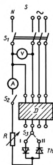
S — источник электрической энергии; I — независимая линия питания; V — вольтметр; A — амперметр (показывающий истинное действующее значение); D — УЗО — Д, подвергаемое испытанию; R — регулируемый резистор; S_1 — многополюсный выключатель; S_2 — однополюсный выключатель; S_3 — двухполюсный выключатель на два направления; S_4 — вспомогательный выключатель; Th — тиристоры
