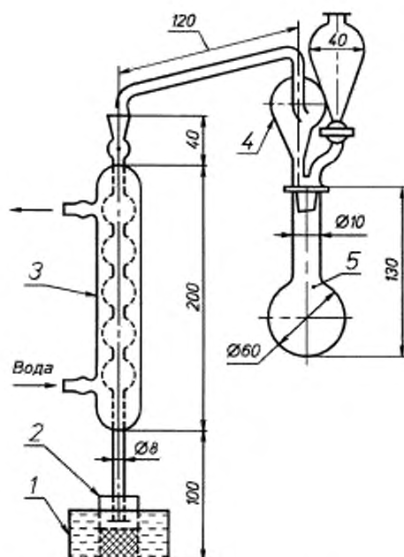
1 — сосуд с холодной водой; 2 — приемник дистиллята; 3 — холодильник; 4 — насадка; 5 — перетонная круглодонная колба
