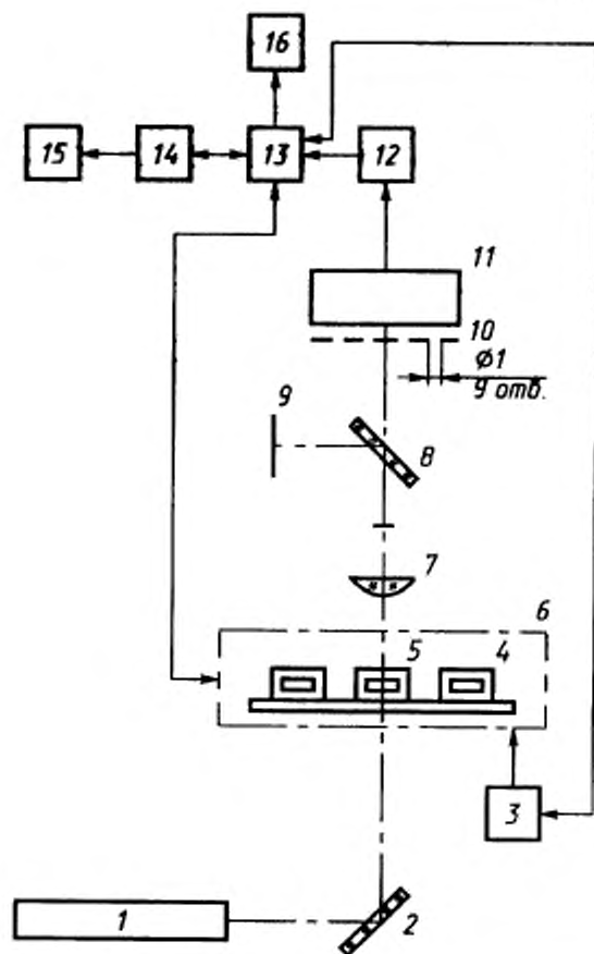
1 — лазер; 2 — светоделительная пластина; 3 — блок термостатирования; 4 — каретка; 5 — капилляр; 6 — привод; 7 — микрообъектив; 8 — светоделительная пластина; 9 — экран; 10 — маска; 11 — фотодиод; 12 — усилитель; 13 — контроллер; 14 — компьютер; 15 — принтер; 16 — блок подготовки проб и рабочих образцов.
