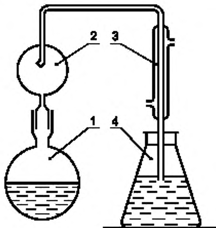
1 - круглодонная колба, 2 - каплеуловитель, 3 - холодильник, 4 - приемная колба
