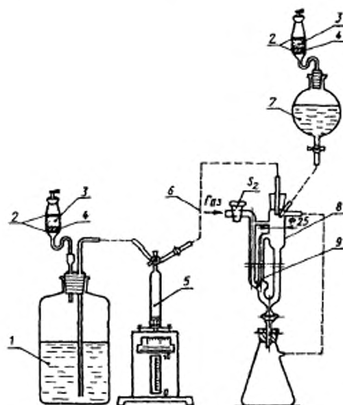
1 — титрант, 2 — стекловолокно, 3 — кран, 4 — ангидрон, 5 — бюретка с поршнем, 6 — соединительная трубка из поливинилхлорида, 7 — пиридин, 8 — поглотительный сосуд, 9 — кинкшпир диаметром 1 мм
