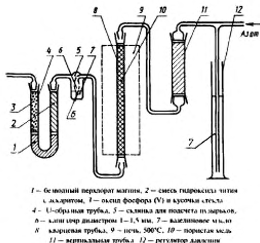
Рисунок 6 — Устройство для очистки азота
