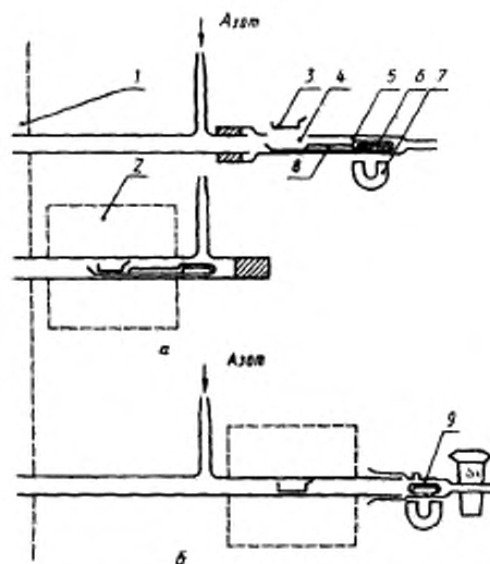
Рисунок 7 — Типичные конструкции входного отверстия трубки для пиролиза
