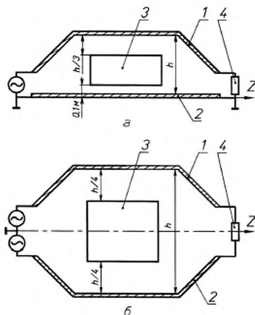
а — преобразователь с несимметричным питанием: 1, 2 — электроды, образующие линию (1 — электрод с нулевым потенциалом), 3 — рабочий объем, 4 — нагрузка; б — преобразователь с симметричным питанием: 1, 2 — электроды, образующие линию, 3 — рабочий объем, 4 — нагрузка
