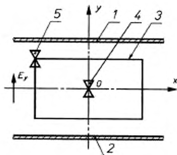
1, 2 — электроды преобразователя; 3 — рабочий объем; 4 — ДАД в центре рабочего объема; 5 — ДАД в одной из вершин параллелепипеда, ограничивающего рабочий объем; O — центр рабочего объема; E_y — вектор напряженности электрического поля в системе координат XYZ; ось Z направлена от плоскости чертежа и совпадает с направлением распространения волны
