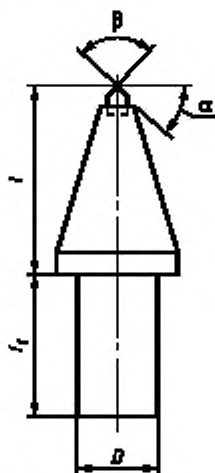
Рисунок 3 — Резец исполнения ТП
