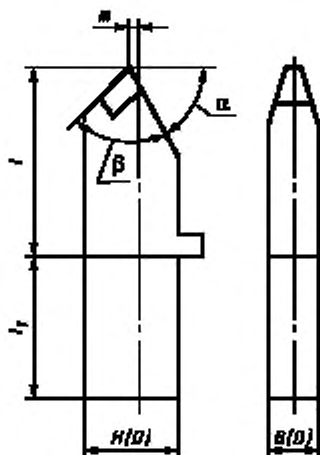
Рисунок 2 — Резец исполнения ТН
