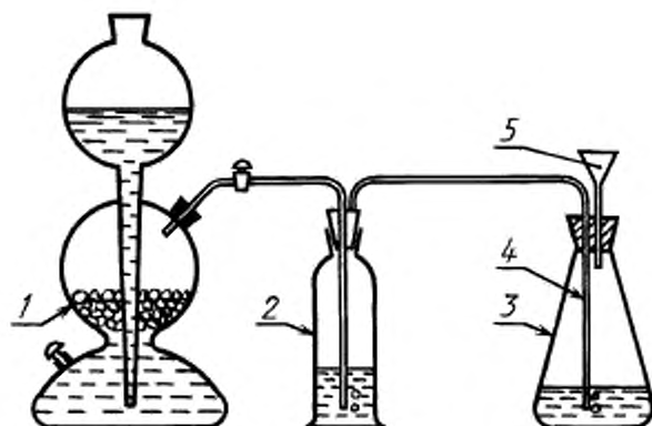
1 — аппарат Киппа для получения углекислого газа (заряжают кусками мрамора и раствором соляной кислоты 1 : 1); 2 — склянка Дрекслея, заполненная раствором сернистой меди; 3 — коническая колба вместимостью 500 см 3 ; 4 — отводная трубка, 5 — воронка
