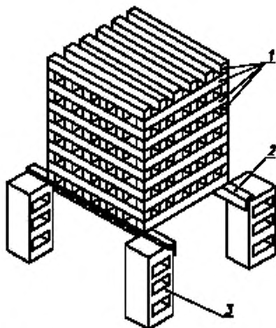
Рисунок А.1 — Устройство деревянного штабеля (модельного очага) для проведения испытаний по тушению пожара класса А
