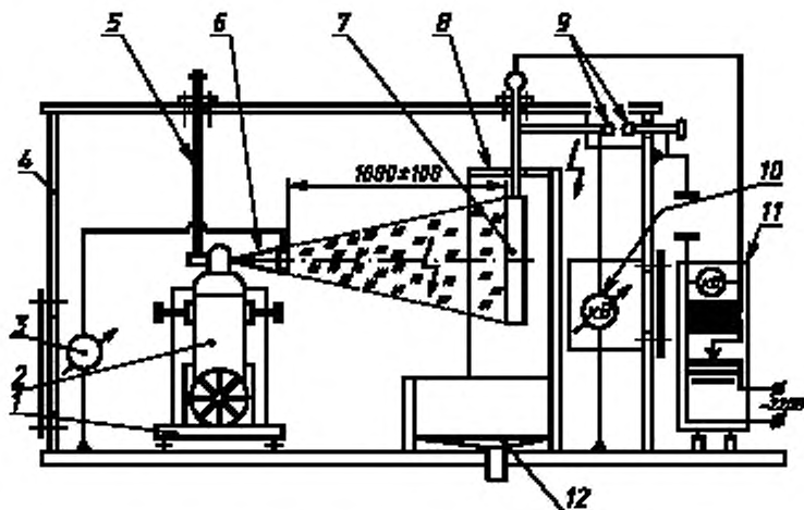
1 — изолирующая подставка; 2 — испытываемый огнетушитель; 3 — измеритель тока утечки; 4 — защитный каркас испытательного стенда; 5 — устройство запуска огнетушителя; 6 — выпускной раструб огнетушителя с электропроводным элементом; 7 — мишень; 8 — экран; 9 — разрядник; 10 — киловольтметр; 11 — источник высокого напряжения; 12 — емкость для сбора обработанного ОТВ
