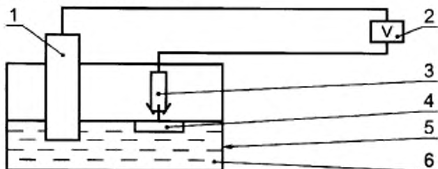
1 — стандартный электрод (хлорсеребряный ЭВЛ-1М3 или платиновый ЭТПЛ-01М); 2 — высокоомный вольтметр с погрешностью измерения \pm 10\% ; 3 — зажим типа «крокодиль»; 4 — протезы с покрытием; 5 — стеклянный стакан или электрохимическая ванночка; 6 — модельная среда (см. 5.6.1)
