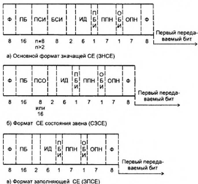
Рисунок 8.2 — Форматы сигнальных единиц
