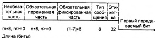
Рисунок 9.3 — Формат сообщений ПУСС
