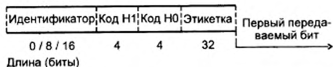
Рисунок 9.4 — Формат сообщений управления сетью сигнализации
