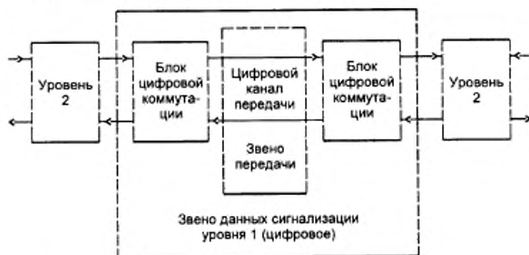
Рисунок 7.1 — Функциональная конфигурация звена данных сигнализации
