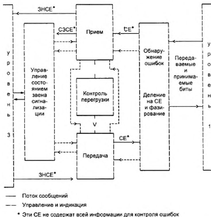
Рисунок 8.1 — Функциональная схема взаимодействия блоков звена сигнализации
