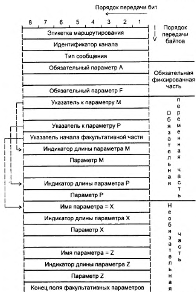
Рисунок 10.1 — Структура сообщения пользователя ЦСИС
