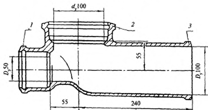
1 — раструб типа I ; 2 — раструб типа IV; 3 — хвостовик
