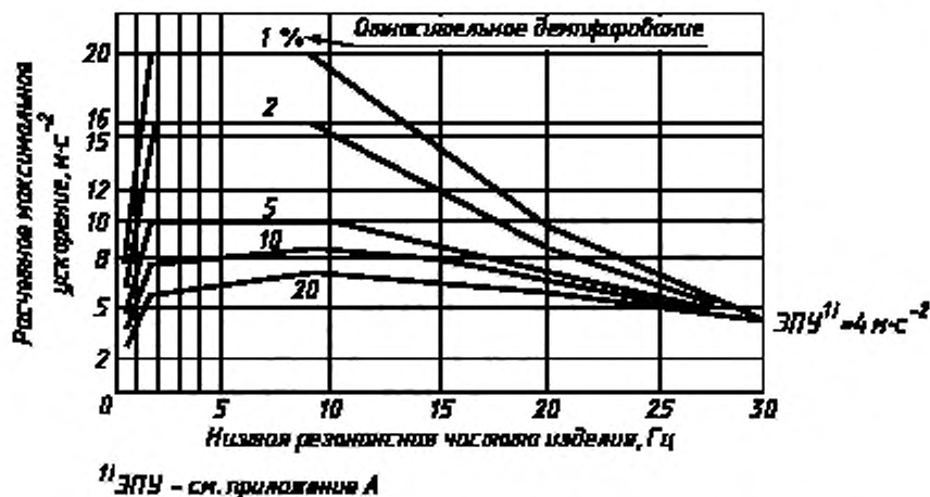
Рисунок 2 — Обобщенные спектры ответа (горизонтальное направление, 9 баллов по MSK — 64 [1])
