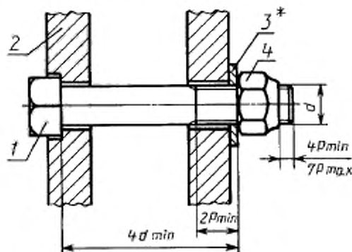
Устройство для измерения усилия затяжки
