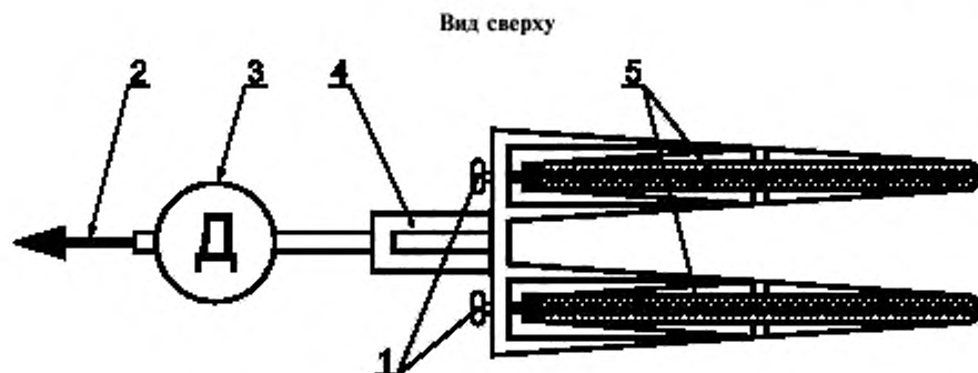
1 — тормоз; 2 — направление движения; 3 — динамометр; 4 — устройство; 5 — колеса
