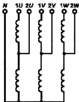
Рисунок Ж.7 — Маркировка трехфазного автотрансформатора ( Y_H\text{ авто}/D-0 )
