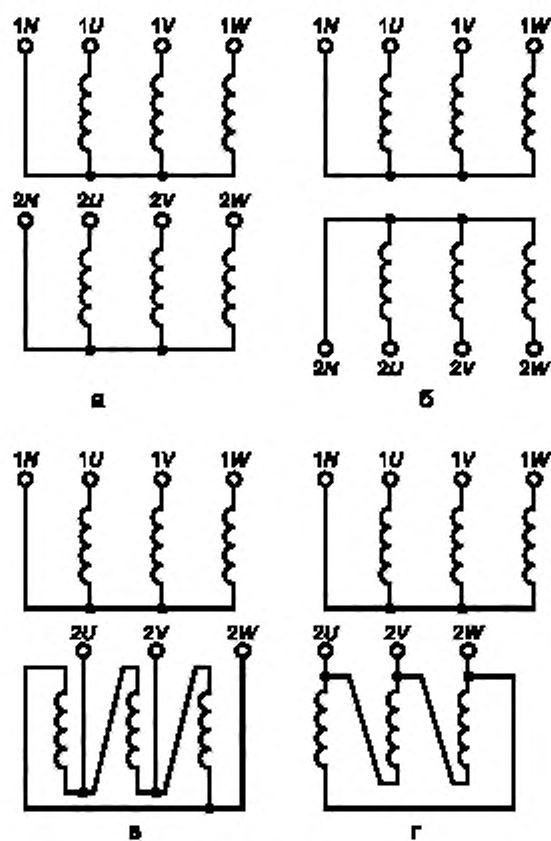
Рисунок Ж.4 — Маркировка трехфазных двухобмоточных трансформаторов
