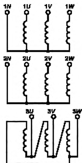
Рисунок Ж.5 — Маркировка трехфазного трехобмоточного трансформатора ( Y_H/Y_H/D-0-5 )
