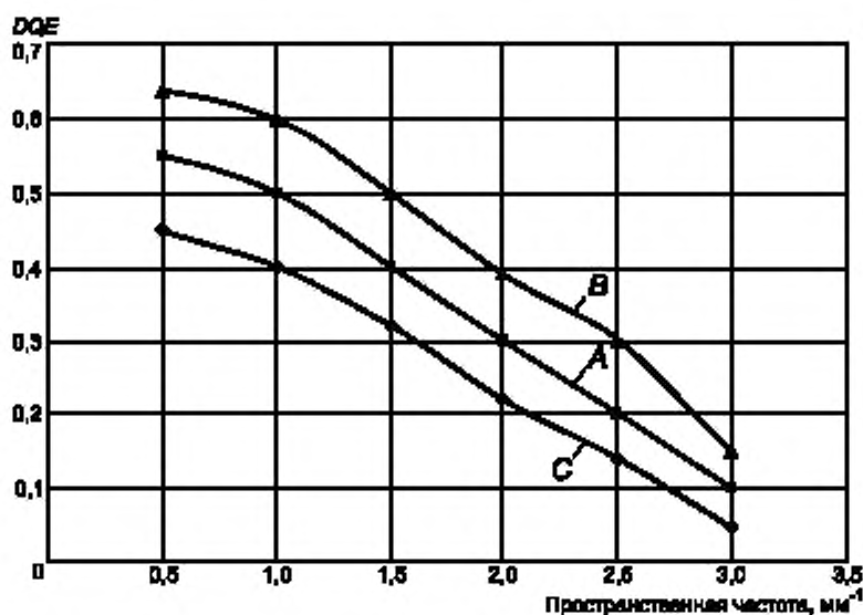
Рисунок 4 — Зависимость DQE от ПРОСТРАНСТВЕННОЙ ЧАСТОТЫ при значениях дозы A: 2,5 мкГр; B: 2,5 мкГр/3,2; C: 2,5 мкГр/3,2
