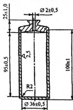
Рисунок 3 — Пикнометр
