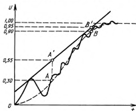
Рисунок 11 — Допустимые колебания на фронте импульса
