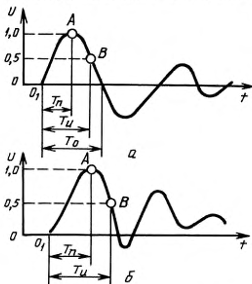
Рисунок 14 — Колебательный коммутационный импульс
