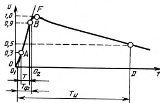
Рисунок 7 — Полный грозовой импульс
