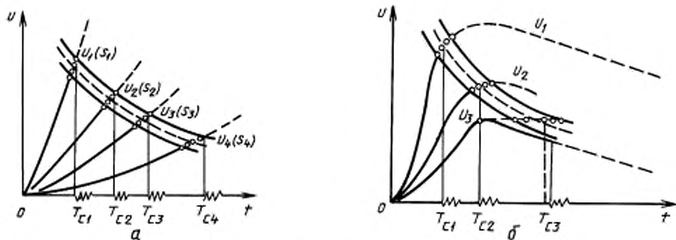
Рисунок 12 — Вольт-секундные характеристики
