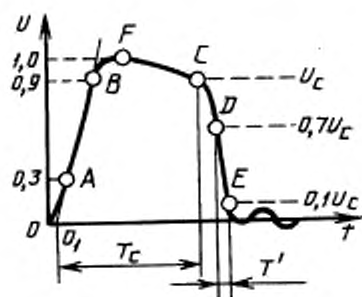
Рисунок 9 — Грозовой импульс, срезаемый на спаде импульса
