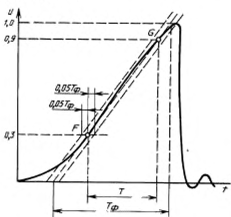
Рисунок 10 — Линейно нарастающий импульс
