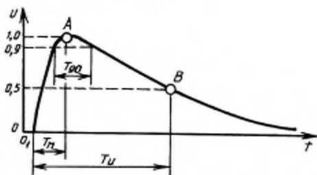
Рисунок 13 — Апериодический коммутационный импульс
