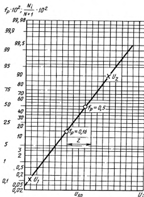
Рисунок А.1 — Вероятностная сетка
