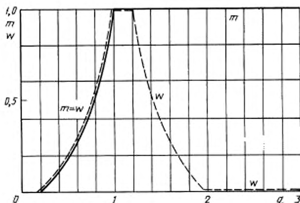
Рисунок 5 — Показатели степени m и w
