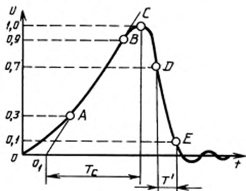
Рисунок 8 — Грозовой импульс, срезанный на фронте
