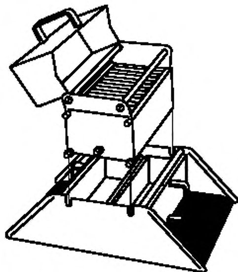
Рисунок А.2 — Множественно-щелевой делитель с системой сортировки
