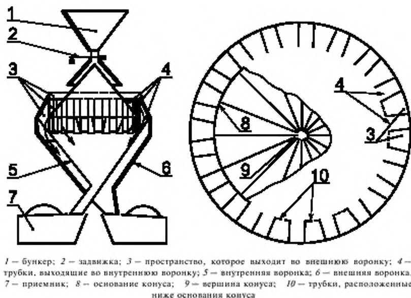
Рисунок А.1 — Конический делитель
