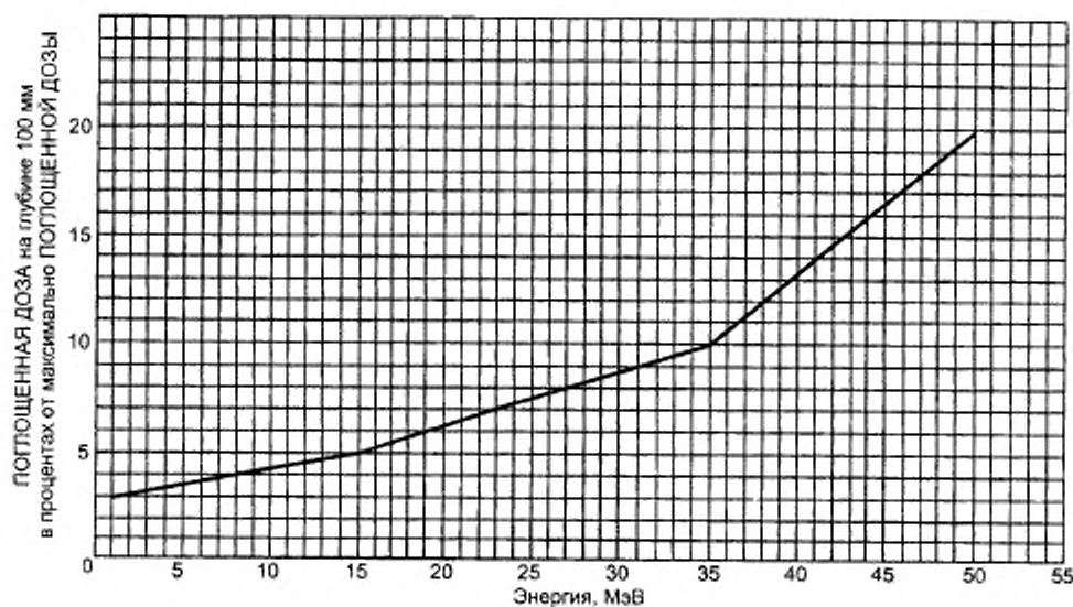
Рисунок 101 — Пределы НЕИСПОЛЪЗУЕМОГО ТОРМОЗНОГО ИЗЛУЧЕНИЯ во время ЭЛЕКТРОННОГО ОБЛУЧЕНИЯ (29.2.1)
