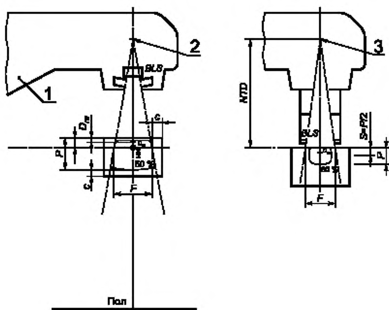
1 – ШТАТИВ; 2 – виртуальный источник ТОРМОЗНОГО ИЗЛУЧЕНИЯ; 3 – виртуальный источник ЭЛЕКТРОННОГО ИЗЛУЧЕНИЯ; \Phi – ИЗОЦЕНТР; S – стандартная измерительная глубина; P – величина, характеризующая качество проникающего ИЗЛУЧЕНИЯ; C – часть ФАНТОМА, изнутри примыкающая к его граничным плоскостям; D_m – максимальное значение глубины дозы на ОСИ ПУЧКА ИЗЛУЧЕНИЯ; BLS – система коллимирования ПУЧКА ИЗЛУЧЕНИЯ; F – размер ПОЛЯ ОБЛУЧЕНИЯ; NTD – нормальное расстояние ОБЛУЧЕНИЯ
