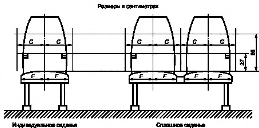
Рисунок 3.5 — Ширина пассажирских сидений (см. 5.7.9.1)
