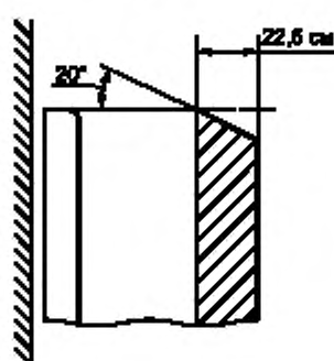
Рисунок 3.15 — Пространство для ног пассажира
