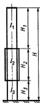
Рисунок 2 — Коэффициенты \beta_i , \beta_k
