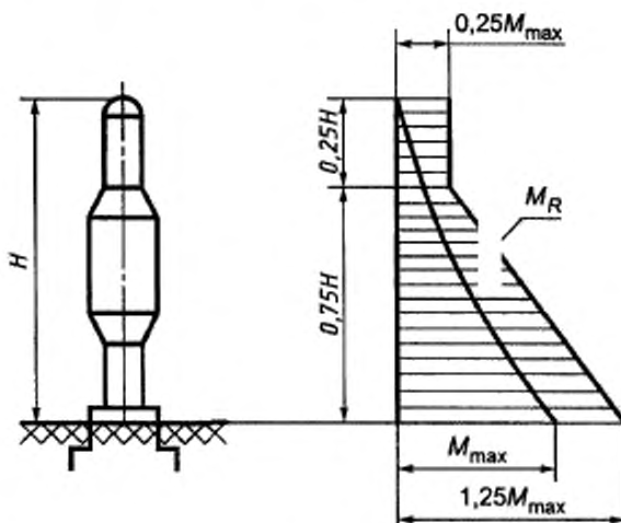
Рисунок 10 — Эпюра для определения изгибающего момента M_R
