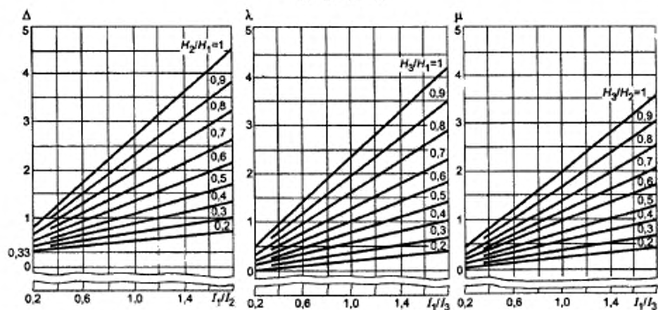
Рисунок 3 — Коэффициенты \Delta , \lambda , \mu
