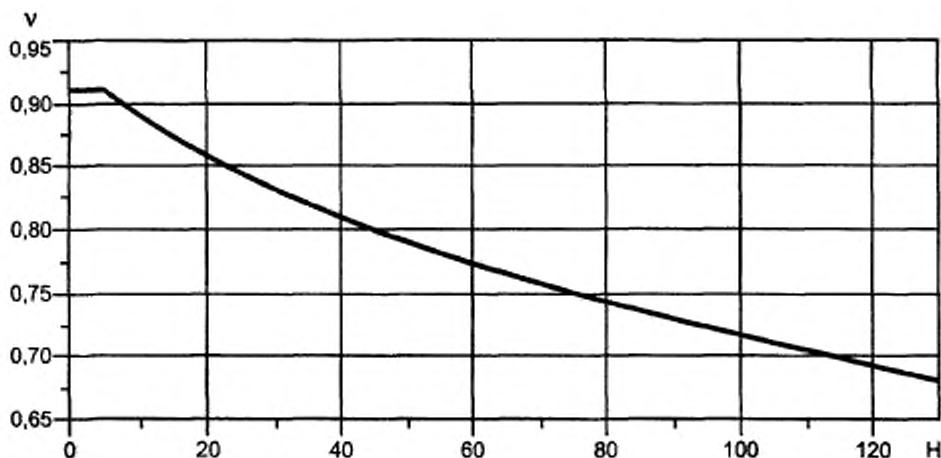
Рисунок 7 — Коэффициент пространственной корреляции пульсаций давления ветра v
