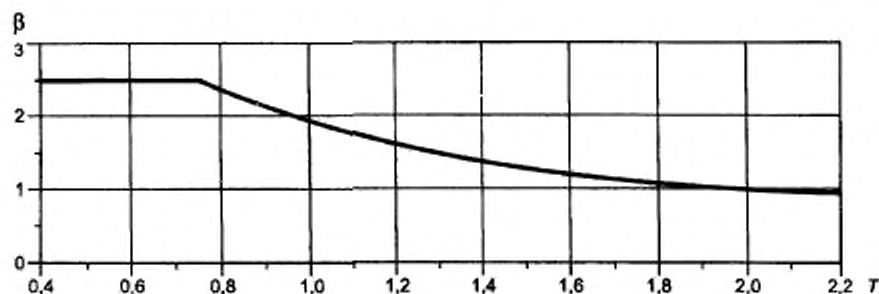
Рисунок 9 — Коэффициент динамичности \beta
