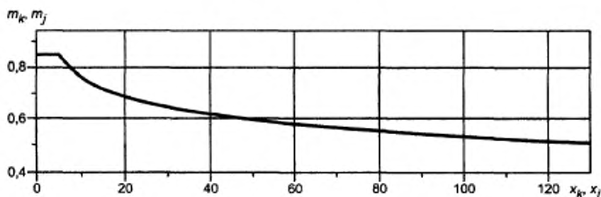
Рисунок 6 — Коэффициенты пульсации давления ветра m_k, m_j
