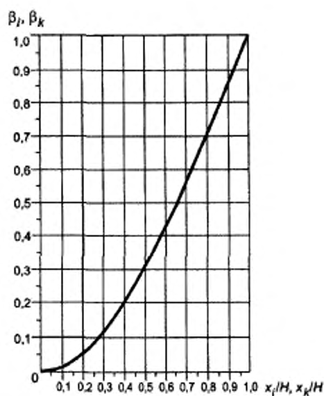
Рисунок 2 — Коэффициенты \beta_i , \beta_k
