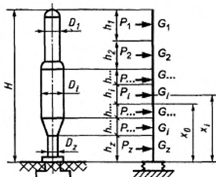
Рисунок 1 — Расчетная схема аппарата
