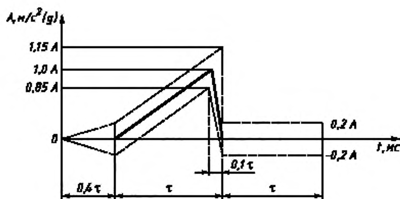
Рисунок А.2 — Треугольный (пилообразный) импульс ударного воздействия
