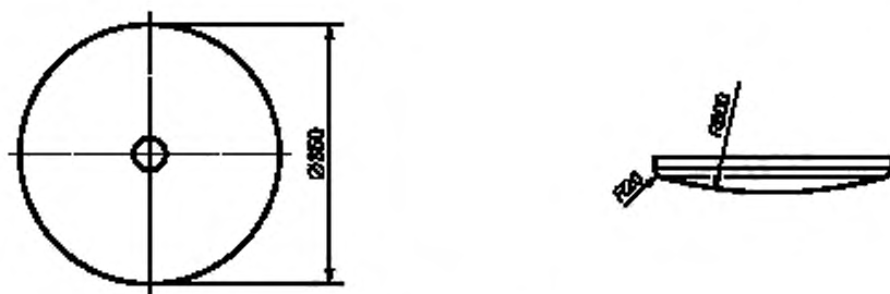
Рисунок ВВ.3 — Подушка с нагрузкой
