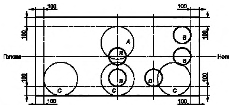
Рисунок ВВ.2 — Положение нагрузок
