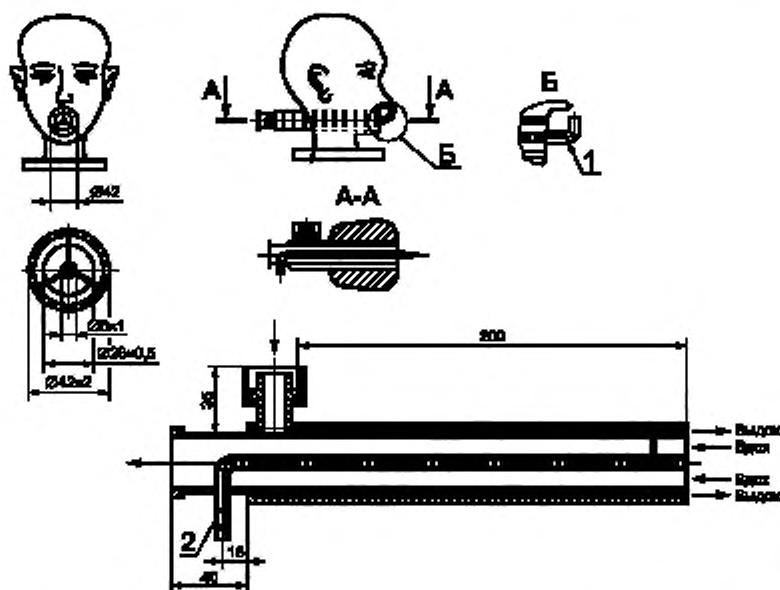
1 — штулка для измерения сопротивления воздушному потоку; 2 — измерение \text{CO}_2
