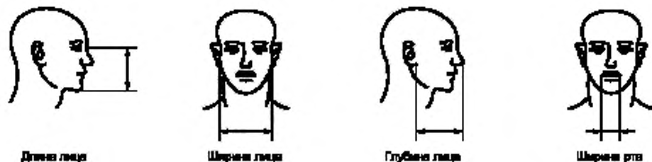
Рисунок 6 — Параметры лица
