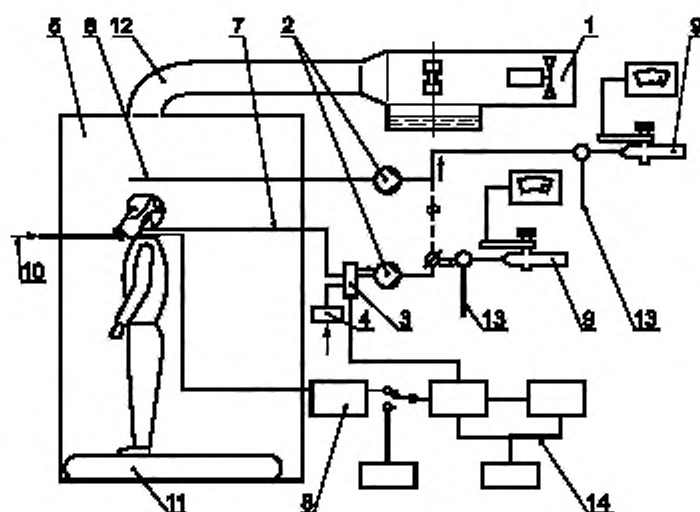
1 — генератор аэрозоля; 2 — насос; 3 — клапан переключения; 4 — фильтр; 5 — испытательная камера (с колпаком); 6 — шланг для отбора проб в испытательной камере; 7 — шланг для отбора проб в подмасочном пространстве; 8 — манометр; 9 — фотометр; 10 — фильтрующая полумаска с клапанами вдоха и несъемными противогазовыми и/или комбинированными фильтрами; 11 — тредбан; 12 — трубопровод и турбулизатор потока; 13 — линия дополнительной подачи воздуха; 14 — система разделения фаз вдоха-выдоха при отборе проб
