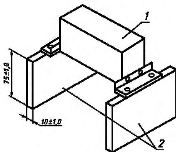
1 — трансформатор; 2 — деревянные подставки
