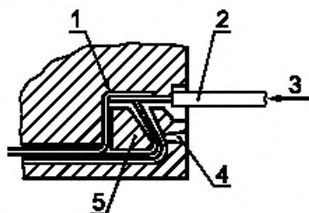
1 — токоведущий проводник; 2 — участок проводника для испытания растягивающим усилием; 3 — проводник, рассчитанный на максимальный ток 3А; 4 — устройство разъединения; 5 — ограничитель
