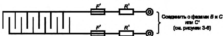
Рисунок Н.3 — Схема соединения решетки
