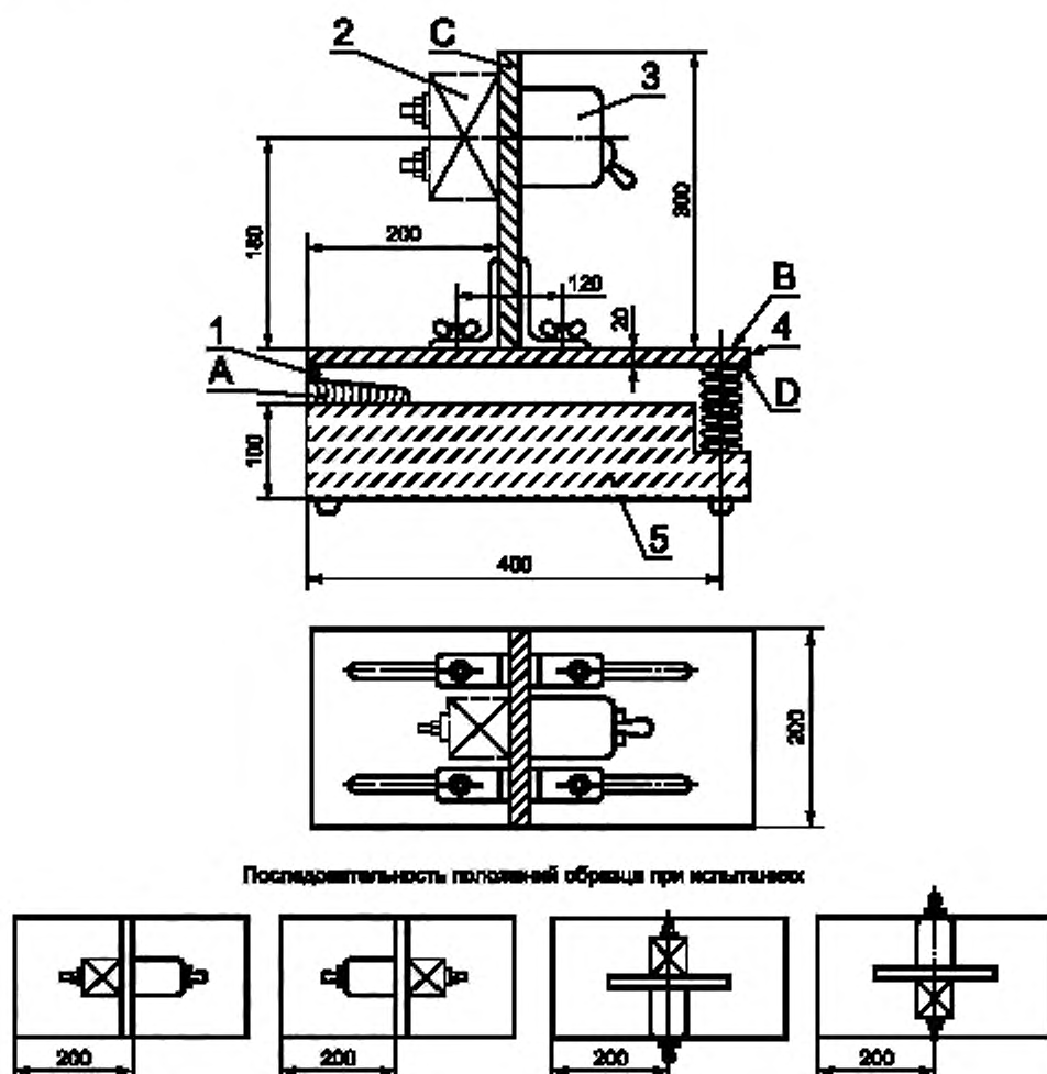
Рисунок 8 — Устройство для испытаний на механические толчки
