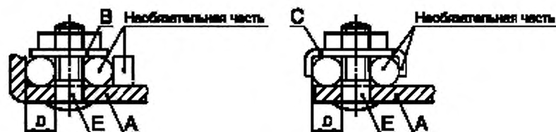
Штыревые выводы
