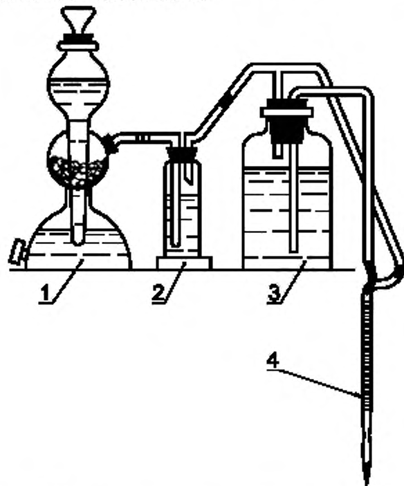
1 — аппарат Киппа; 2 — промывалка для газа, заполненная раствором сернистой соли титана (III) 50 г/дм 3 ; 3 — сосуд с рабочим раствором; 4 — бюретка
