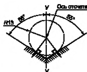
Рисунок 3 — Определение оси отсчета 2)
