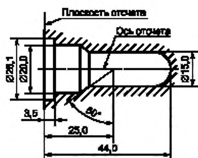
Рисунок 2 — Максимальные размеры лампы 1)
