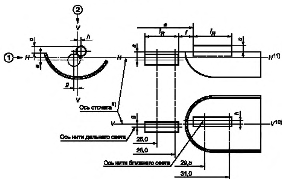
Расположение экранирующей части колбы*
