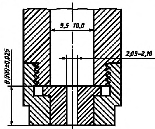
Рисунок 9 — Фильера
