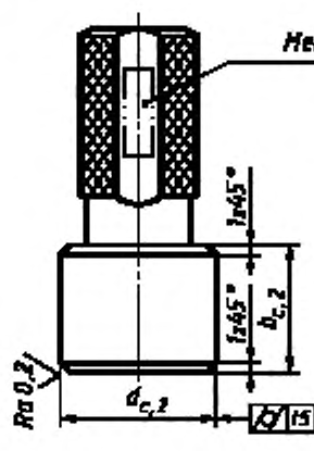
Рисунок 3 — Калибр-пробка сплошная
