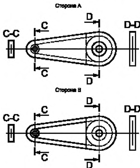
Рисунок 7 — Приводные цепи и защитные устройства цепи
