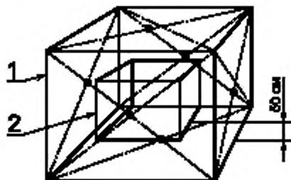
1 — измерительная поверхность (поверхность установки микрофонов); 2 — «боек» размещения игрушки
