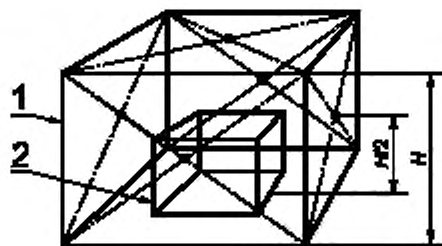
1 — измерительная поверхность (поверхность установки микрофонов); 2 — «боек» размещения игрушки
