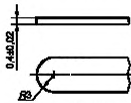
Рисунок 13 — Шуп
