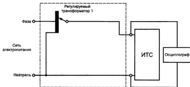
Рисунок Б.2 — Схема устройства для испытаний при воздействии постепенных изменений напряжения
