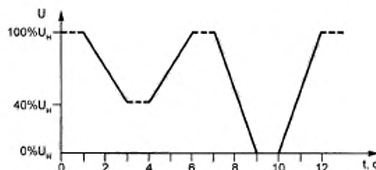
Рисунок 1 — Динамические изменения напряжения (провалы)
