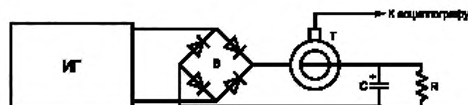
В — выпрямительный мост; Т — токоусъемник с выходом на осциллограф; С — электролитический конденсатор емкостью 1700 мкФ \pm 20\% ; R — резистор не более 10 000 Ом и не менее 100 Ом
