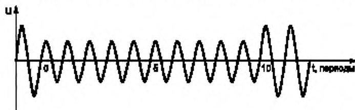
Рисунок 1 — Динамические изменения напряжения (провалы)
