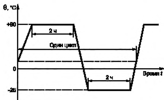
Рисунок F.8 — Цикл испытаний на тепловой удар
