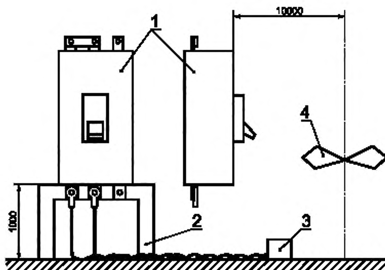
1 — испытуемый выключатель; 2 — изолирующая опора; 3 — источник питания; 4 — антенна
