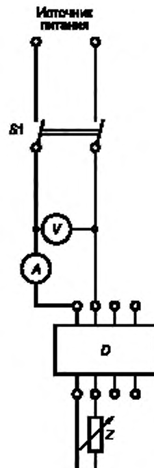
A — амперметр; V — вольтметр; D — испытываемый АВДТ; S1 — двухполюсный выключатель; Z — регулируемое полное сопротивление
