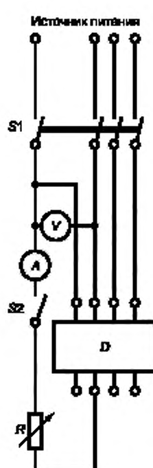
С1 — многополюсный выключатель; S2 — однополюсный выключатель; D — испытываемый АВДТ; V — вольтметр; A — амперметр; R — регулируемый резистор
