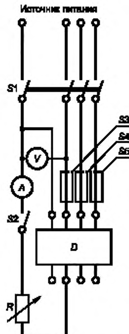
V — вольтметр, A — амперметр; D — испытываемый АВДТ; S1 — многополюсный выключатель; S2 — однополюсный выключатель; S3, S4, S5 — однополюсные выключатели, размыкающие одну фазу (поочередно); R — регулируемый резистор
