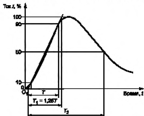
Рисунок В.6 — Волна импульсного тока 8 / 20 мкс
