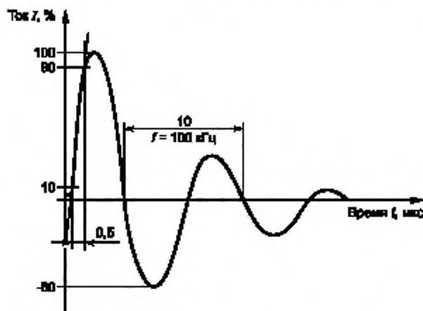
Рисунок В.4 — Волна тока 0,5 мкс / 100 кГц
