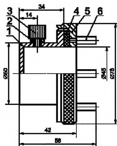
Рисунок 3 — Диффузионная ячейка для испытания гравиметрическим методом
