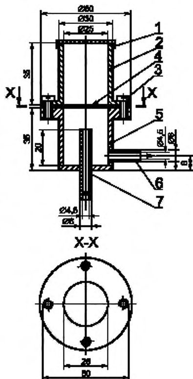
1 — крышка, 2 — верхняя камера, 3 — зажимные болты; 4 — элементарная проба; 5 — нижняя камера; 6 — выходной штуцер; 7 — входной штуцер
