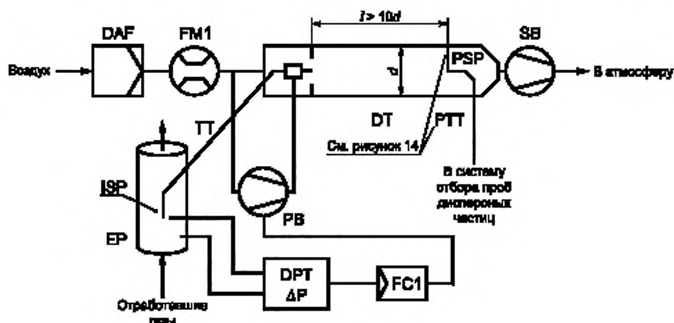
Рисунок 5 — Система разведения части потока с изокINETическим пробоотборником и частичным отбором проб (контроль PB)
