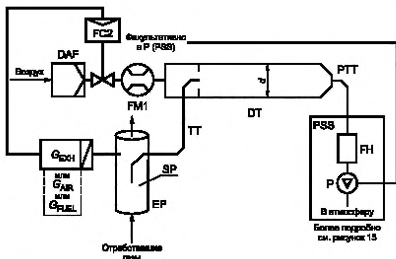
Рисунок 11 — Система разрезания части потока с контролем потока и общим отбором проб
