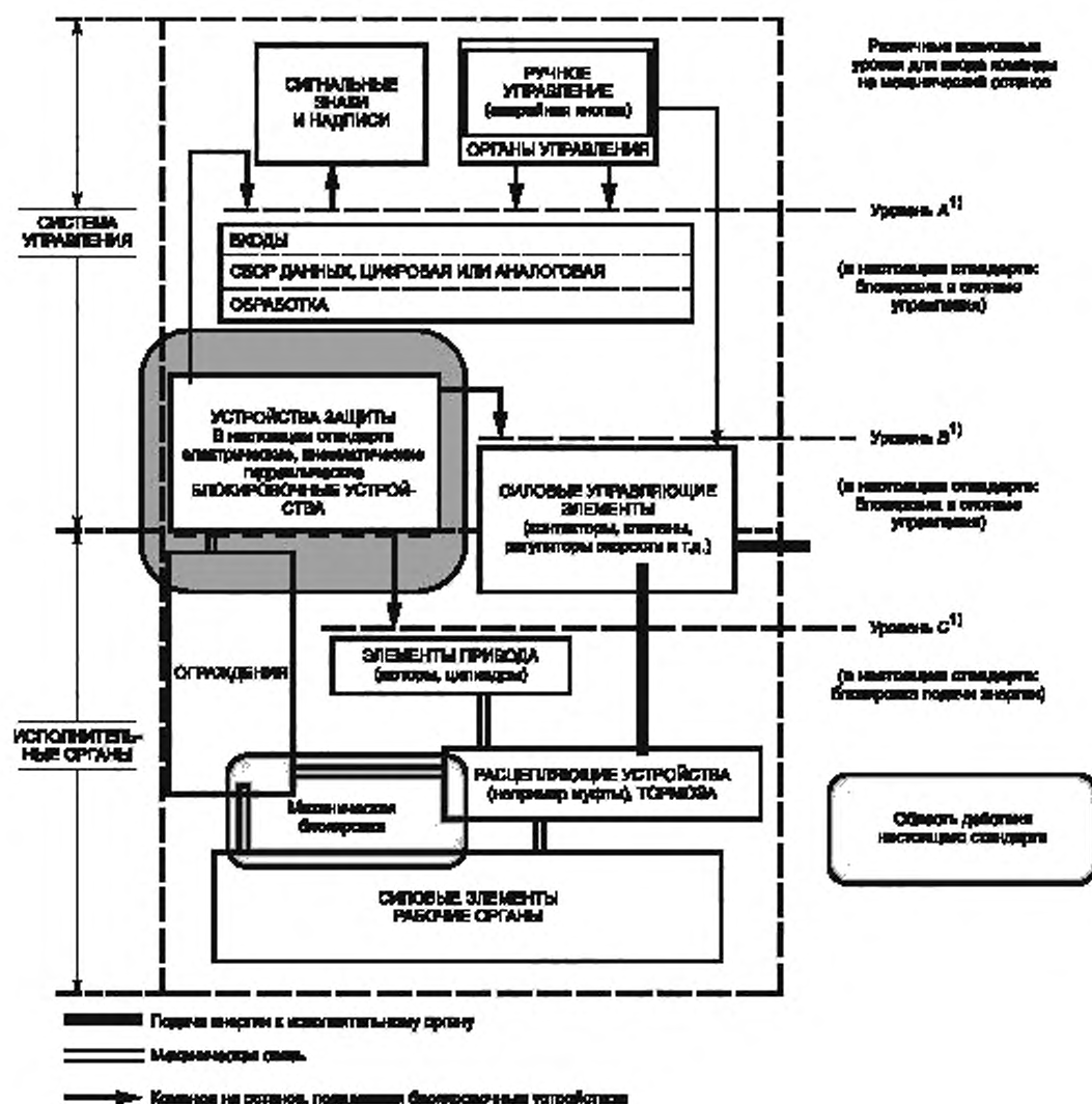
Рисунок 1 — Размещение блокировочных устройств в машинах (ГОСТ Р 51333, приложение А)
