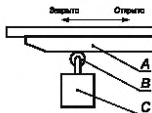
Рисунок А.2 — С поступательно перемещающимся ограждением
