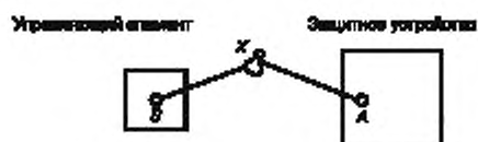
Рисунок Е.1 — Базовая диаграмма блокировочного устройства
