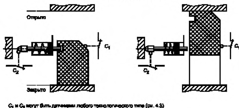
Рисунок М.1 — Раздельные датчики для определения позиции защитного устройства
