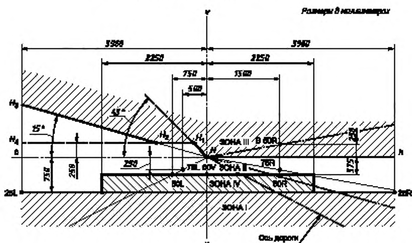
В. Элемент HSB для левостороннего движения
