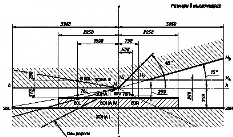
А. Элемент HSB для правостороннего движения
