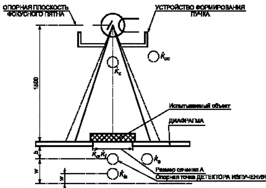
Рисунок 1 — Геометрия ШИРОКОГО ПУЧКА
