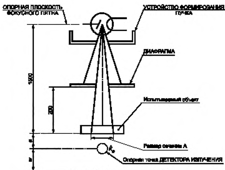
Рисунок 2 — Геометрия УЗКОГО ПУЧКА
